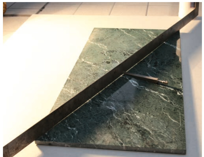
Abb. 9 – Überprüfung der Ebenflächigkeit im Lieferzustand.
